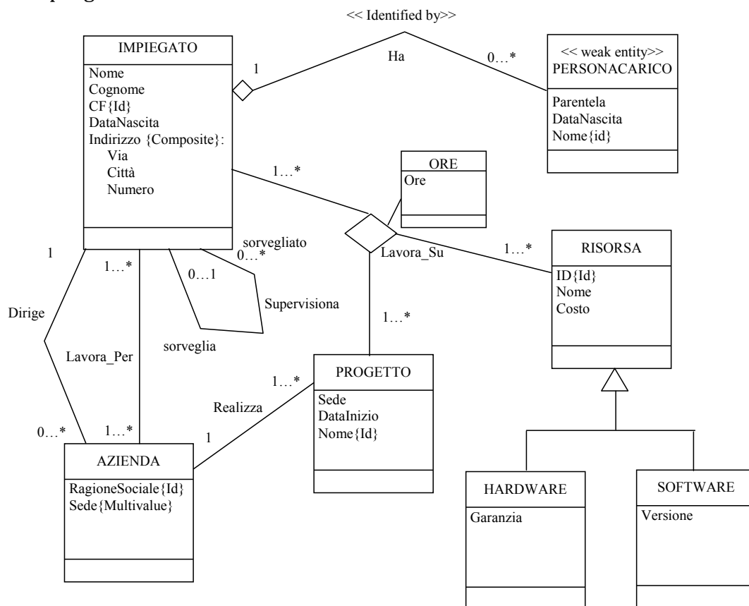
Figure 1: Il class diagram di un sistema per la gestione di una azienda
